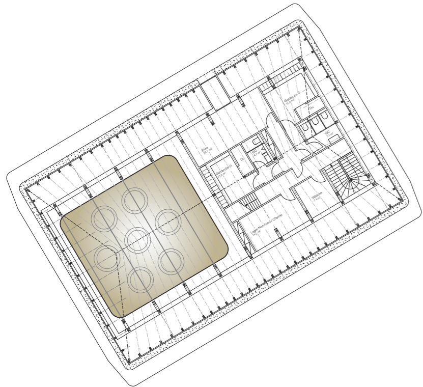
1. Obergeschoss 1 : 100
