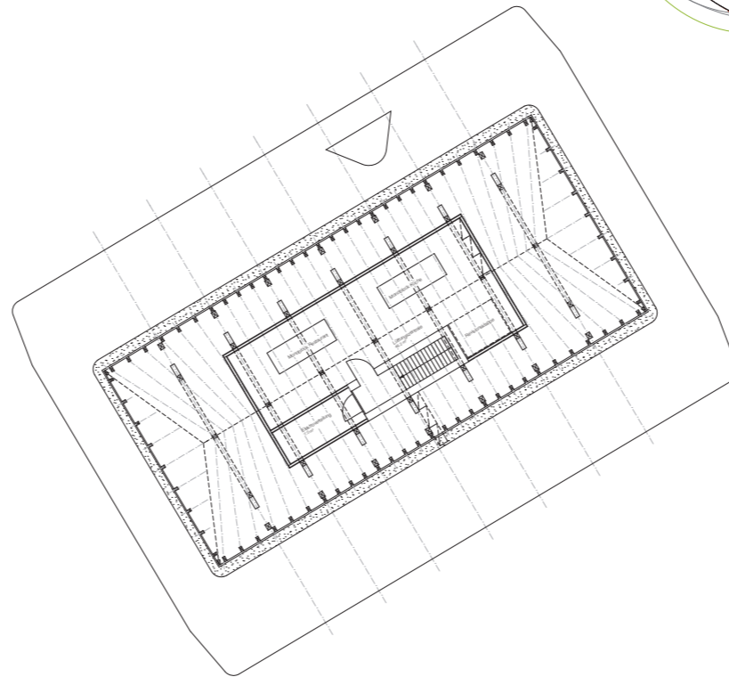
2. Obergeschoss 1 : 100
